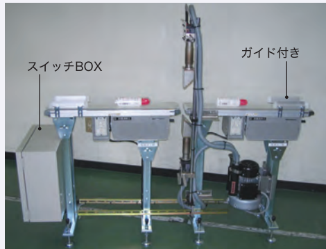
□オーバーフローシュリンク用(上下吹き付けタイプ) 参考価格:900,000円
