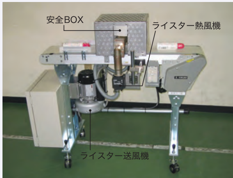
□サイドフローシュリンク用(左右吹き付けタイプ) 参考価格:700,000円
